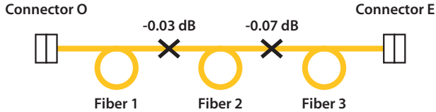
Actual fusion splice loss
